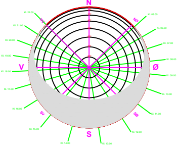
Solens bane 21. juni
